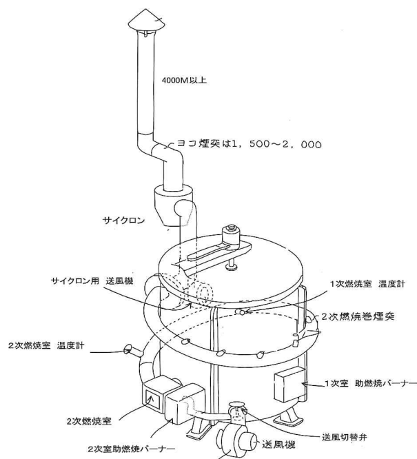
ゴミゼ炉くん CM-20-SOB 型
